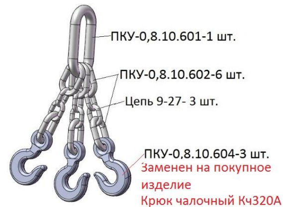
ПКУ-0,8.10.020 Расчалка
