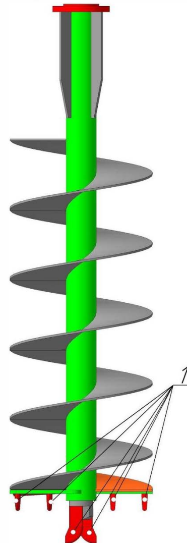
Рисунок 5. Бур НБУ-1300.42
